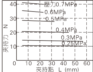
HFTZ20\HFTK20
