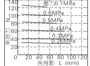
HFSZ32\HFSK32
