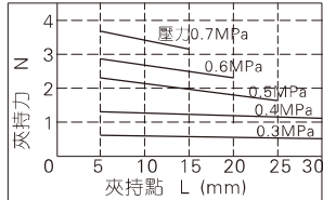
HFTZ10\HFTK10
